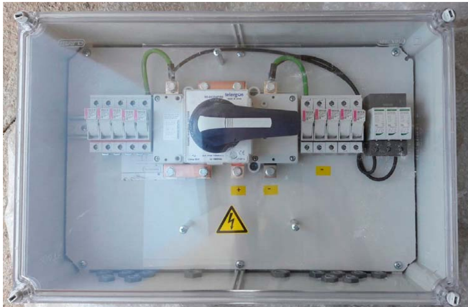
CUADRO STC5 100A
